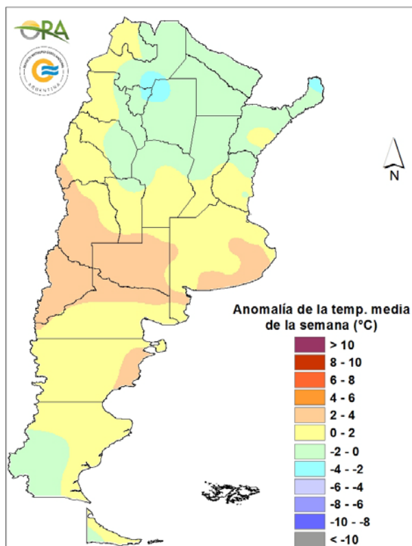
Anomalía de la temperatura media de la semana del 12/11/2025 al 18/11/2025
